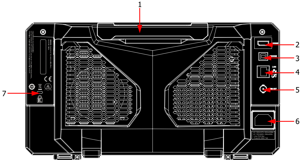
图 1-12 后面板总览
