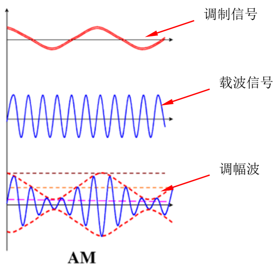
图 17-10 调幅
