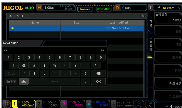
图 18-2 新建目录
