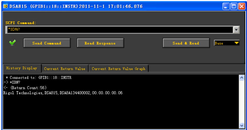
图 3-10 通过 GPIB 读写命令
