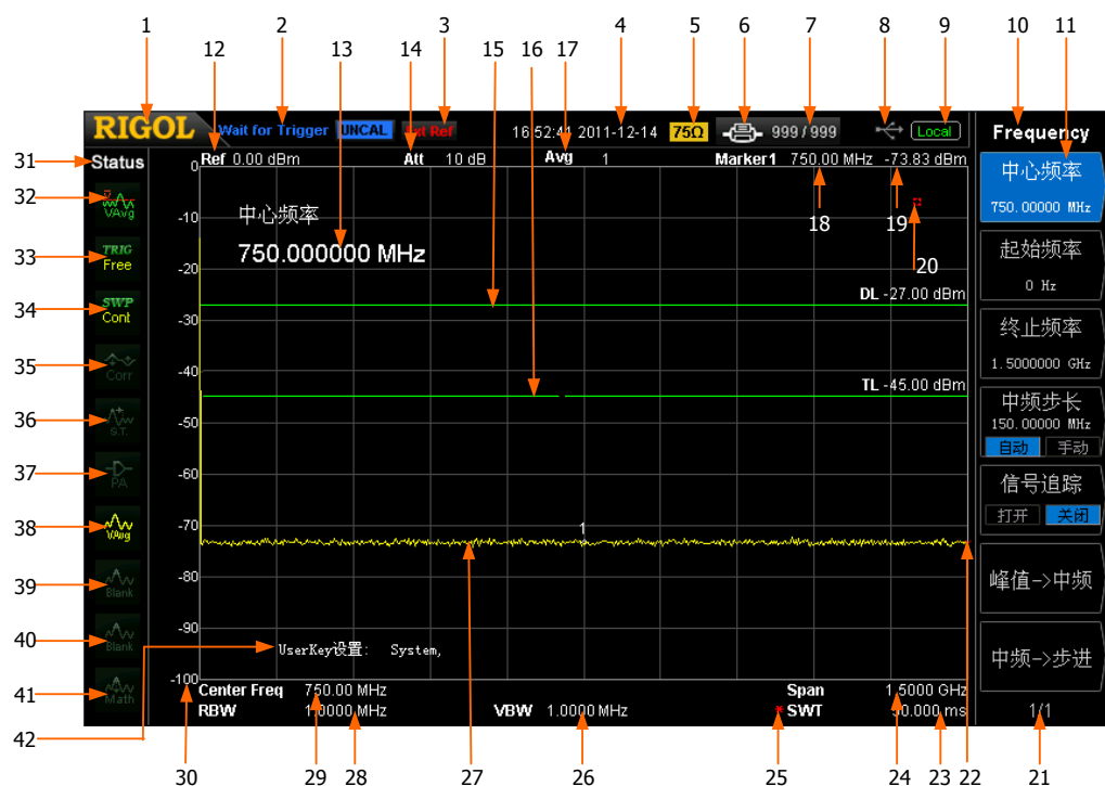
图 1-10 用户界面
