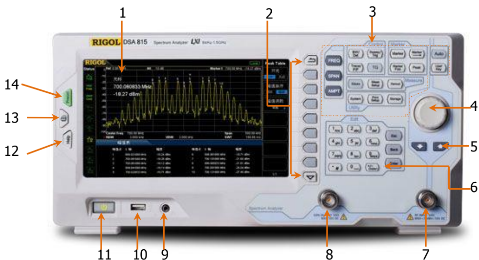
图 1-5 前面板
