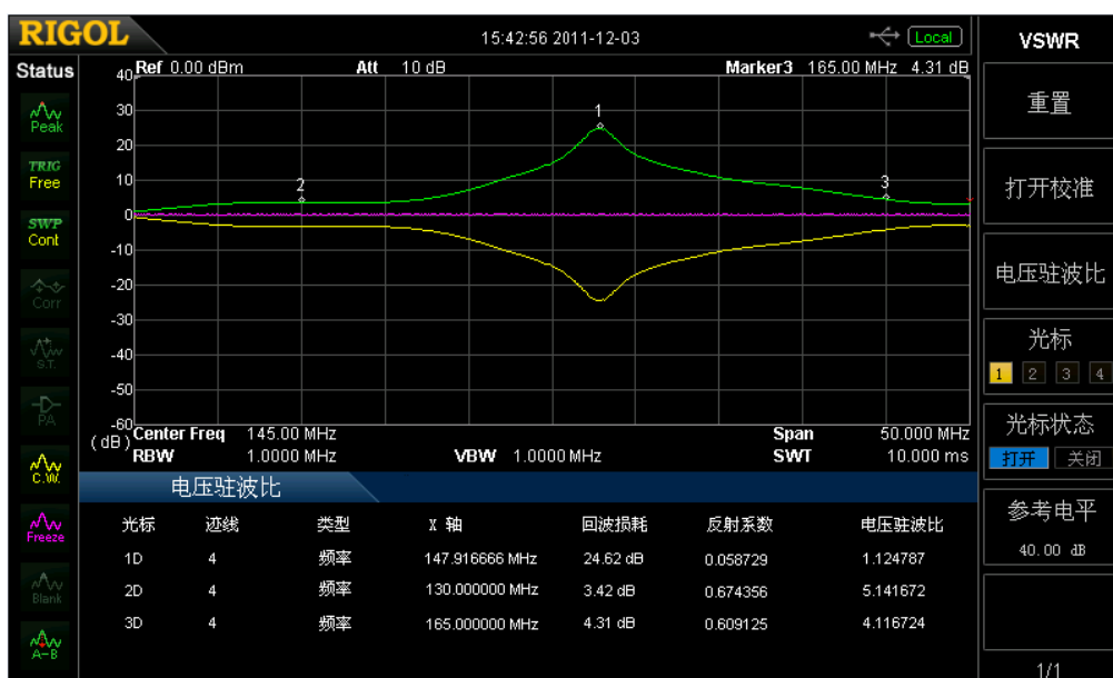
图 2-13 VSWR 测量界面
