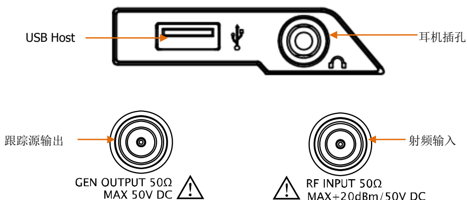
图 1-7 前面板连接器
