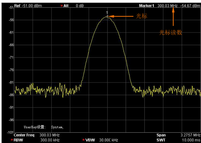
图 2-22 光标示意图
