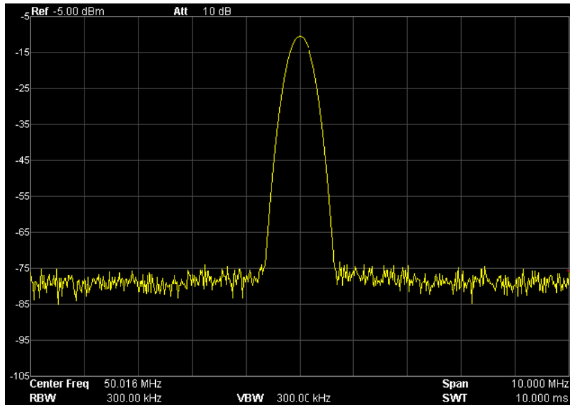
图 2-28 自动搜索信号后
