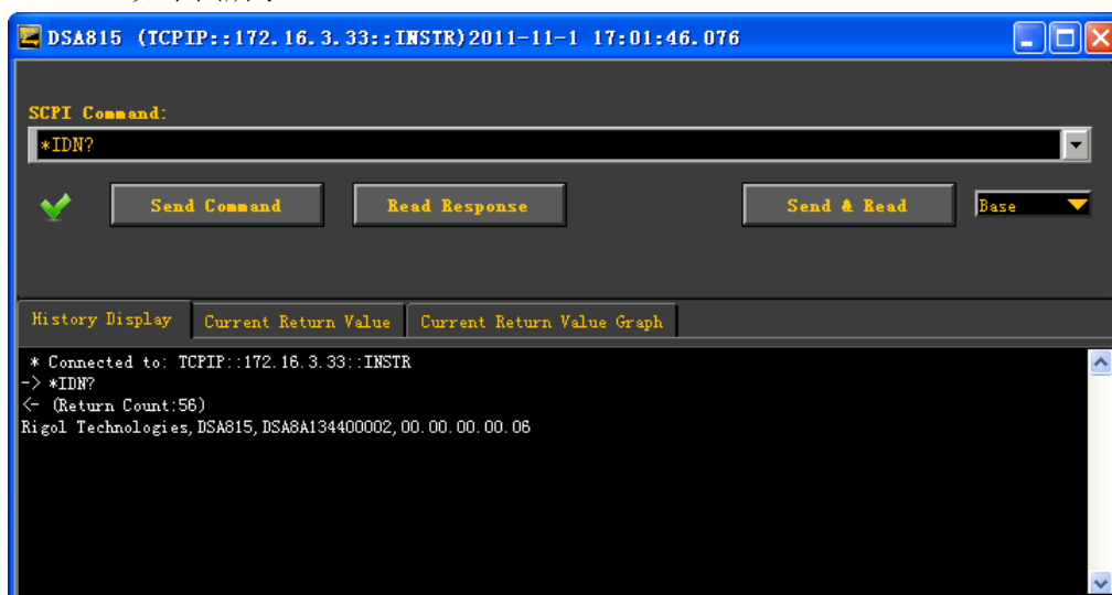
图 3-6 通过 LAN 读写命令
