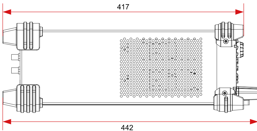
图 1-2 侧视图
