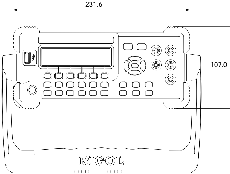
图 1-3 正视图
