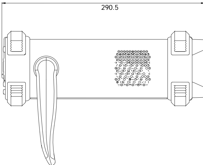
图 1-4 侧视图
