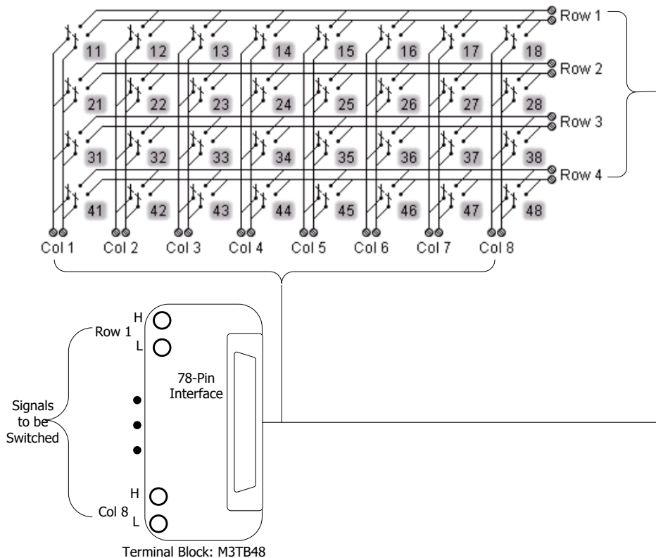
图 2-29 MC3648 示意图
