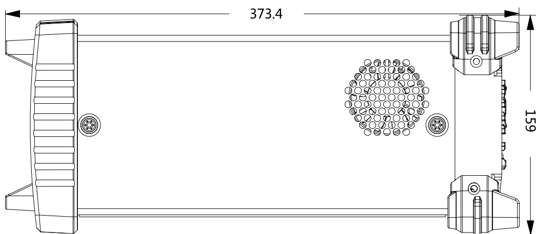
图 1-2 侧视图
