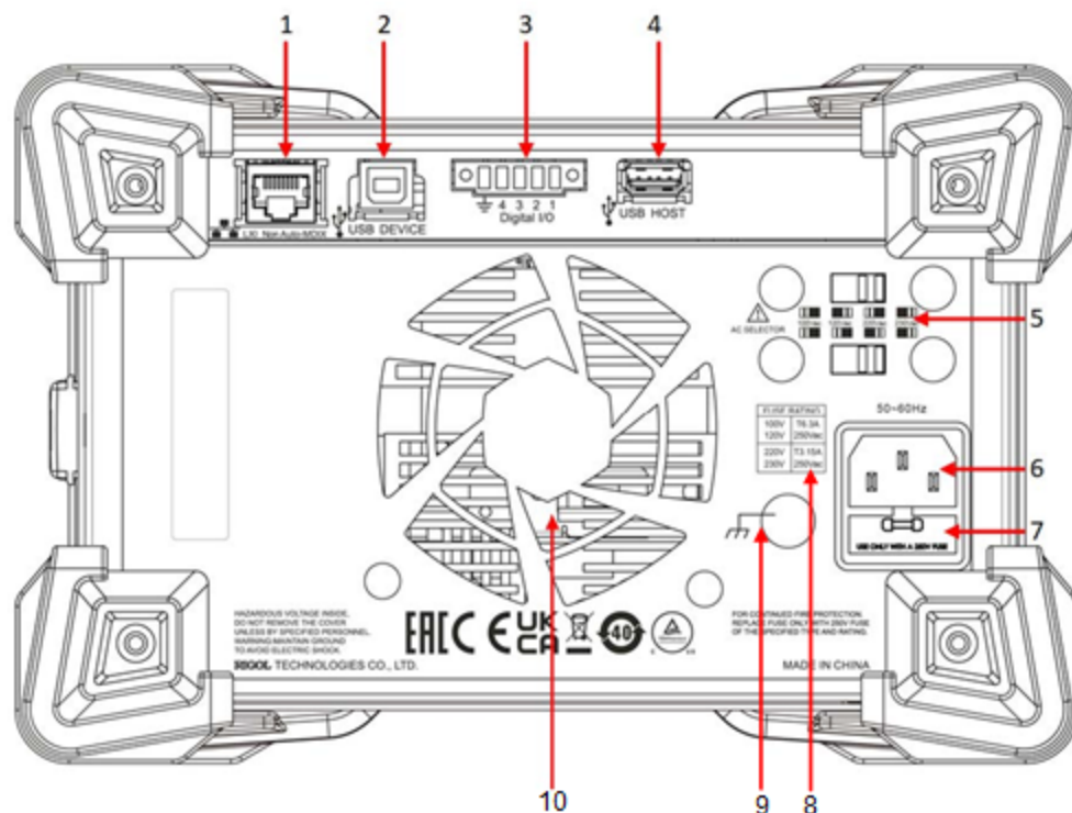
图 4.5 DP900 后面板
