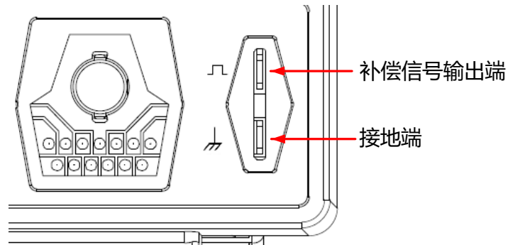
图 4.9 补偿信号
