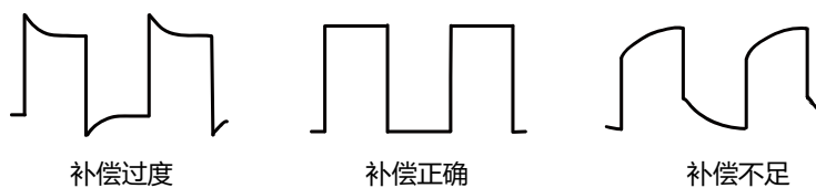
图 4.11 探头补偿
