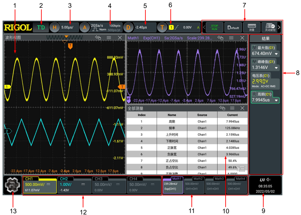
图 4.14 用户界面
