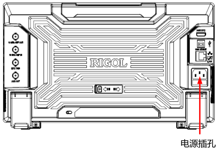
图 4.4 连接电源
