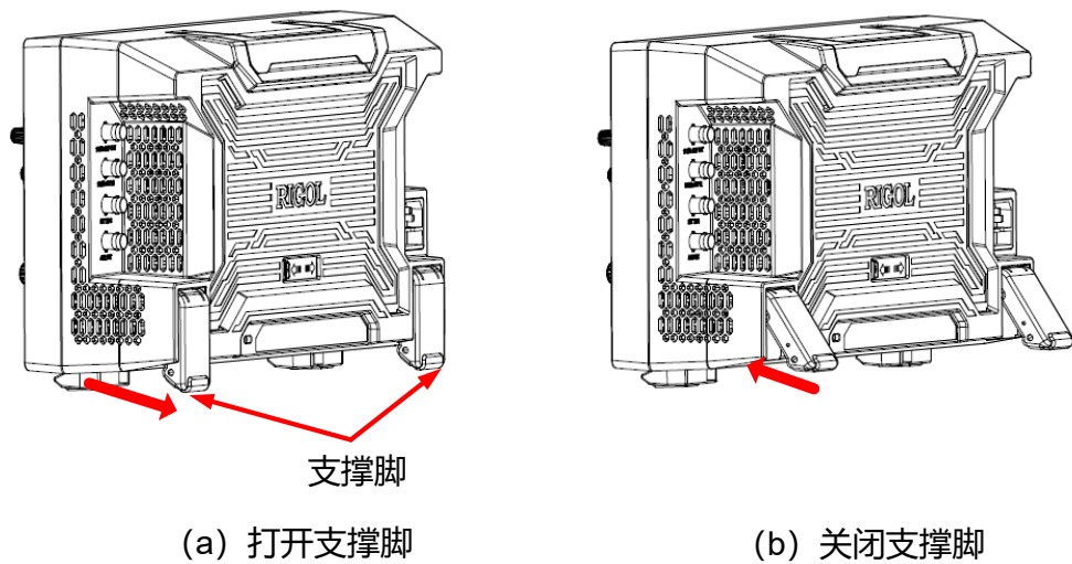
图 4.3 调节支撑脚
