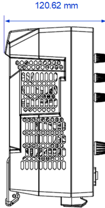
图 4.2 侧视图
