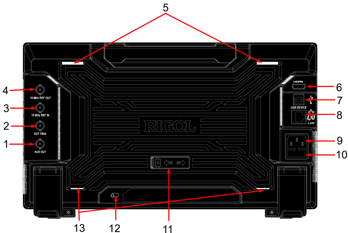
图 4.13 后面板
