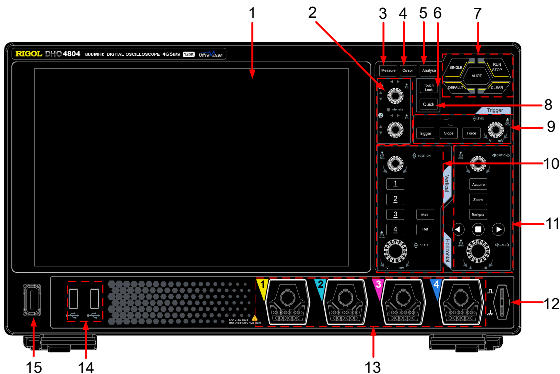
图 4.12 前面板
